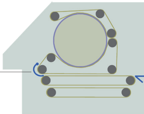
Mechanischer Bypass 1. Längsfaltung
