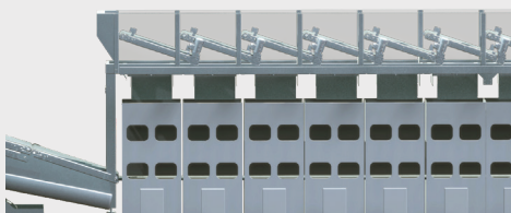
Wiegesilos + Hängebahn
