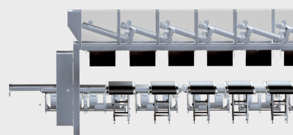
Wiegeförderern + Hängebahn
