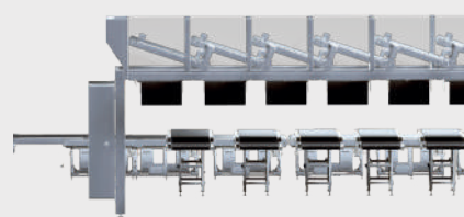
Transportadores de pesagem + Sistema de carga suspensa
